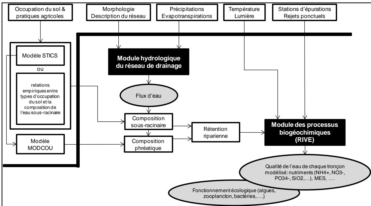
Figure 3.2 : Principes du modèles SENEQUE Ruelland, 2004.
