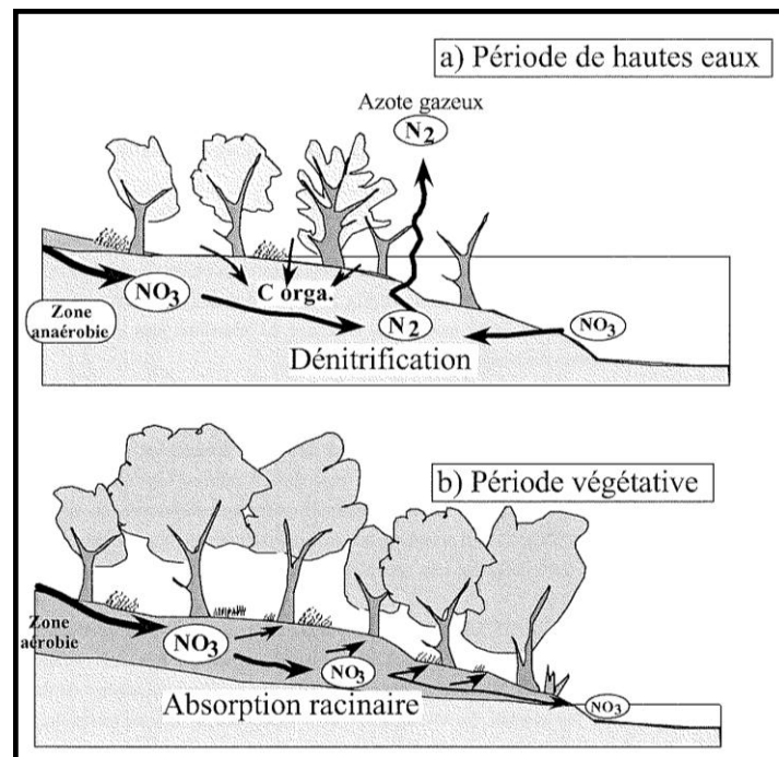
Figure 2.5 : Principaux processus d'épuration des eaux polluées en nitrates par les ripisylves : (a) en période de hautes eaux : dénitration bactérienne anaérobie ; et (b) en période de croissance végétale : absorption racinaire (d'après Maridet, 1995).
