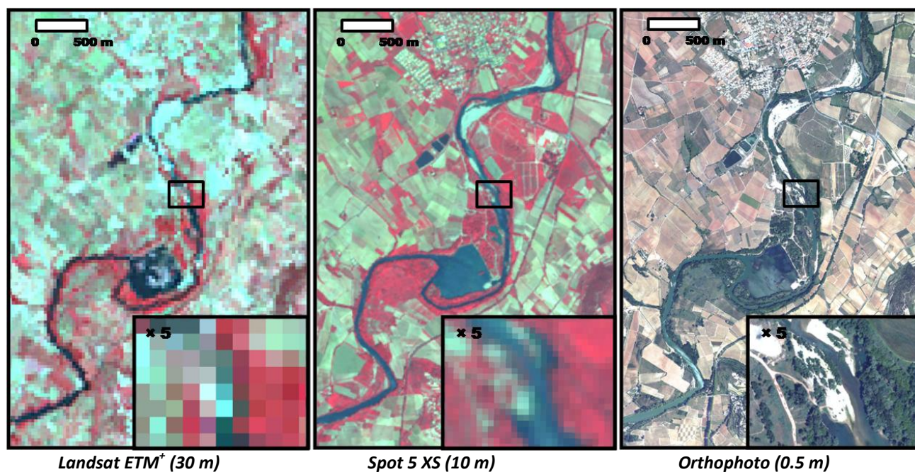
Figure 0.5 : Comparaison d'images à moyenne résolution, Landsat ETM+ (30 m), à haute résolution, Spot 5 XS (10 m) et à très haute résolution spatiale, orthophoto IGN (0.5 m) sur une portion du fleuve Hérault au niveau de sa plaine. L'identification des structures rivulaires est nettement plus visible sur les images à haute et très haute résolution spatiale qui fournissent une information plus riche et plus détaillée.
