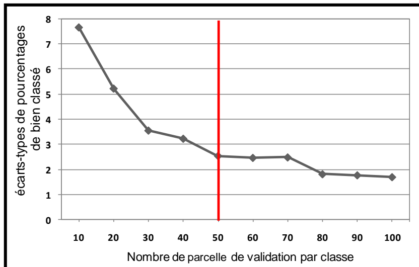
Figure 5.34 : Cette figure présente l'évolution des écarts types de pourcentage d'objets bien classés (précision globale) en fonction de l'augmentation de la taille de l'échantillon de validation.
